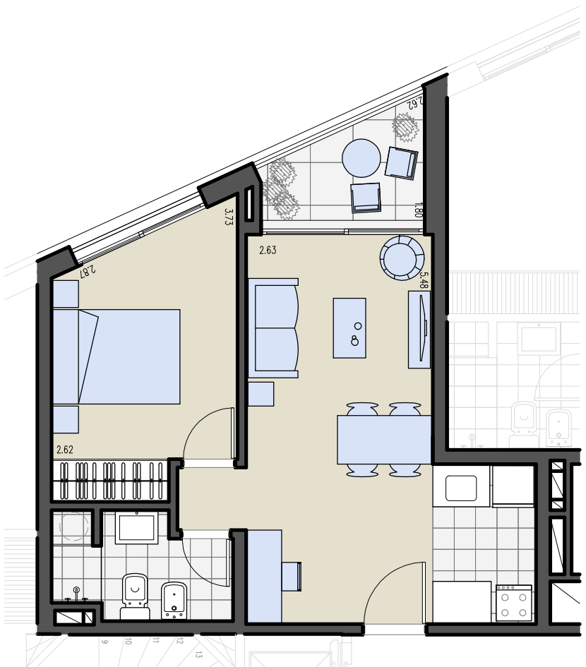
PLANTA UNIDAD 505/905 ESC.1:75
