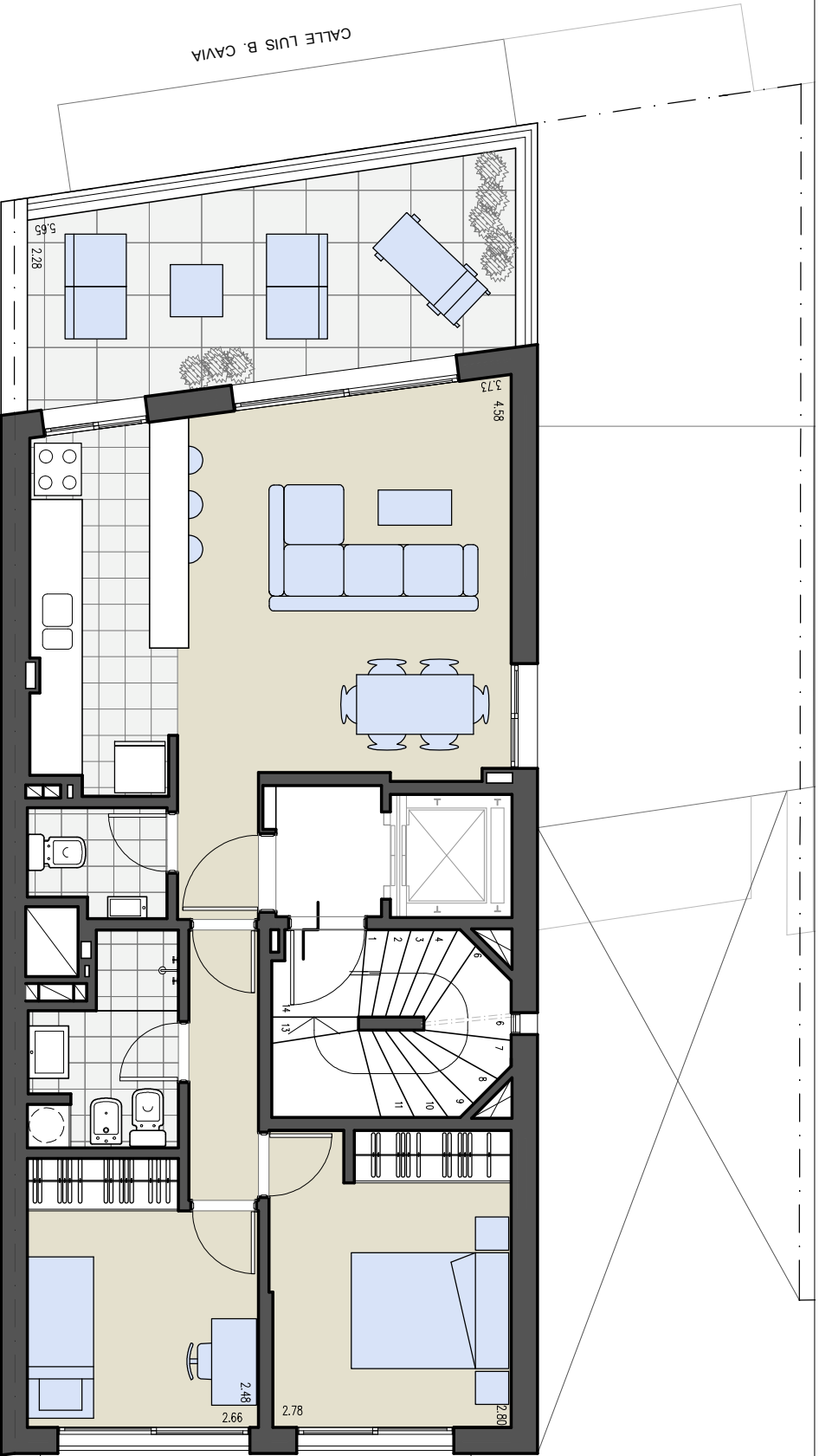
PLANTA UNIDAD 1005 ESC.1:75
